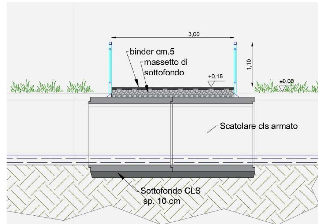
Sezione attraversamento colo
