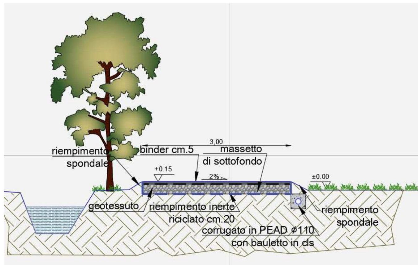
Sezione tipo percorso (tratto 1)
