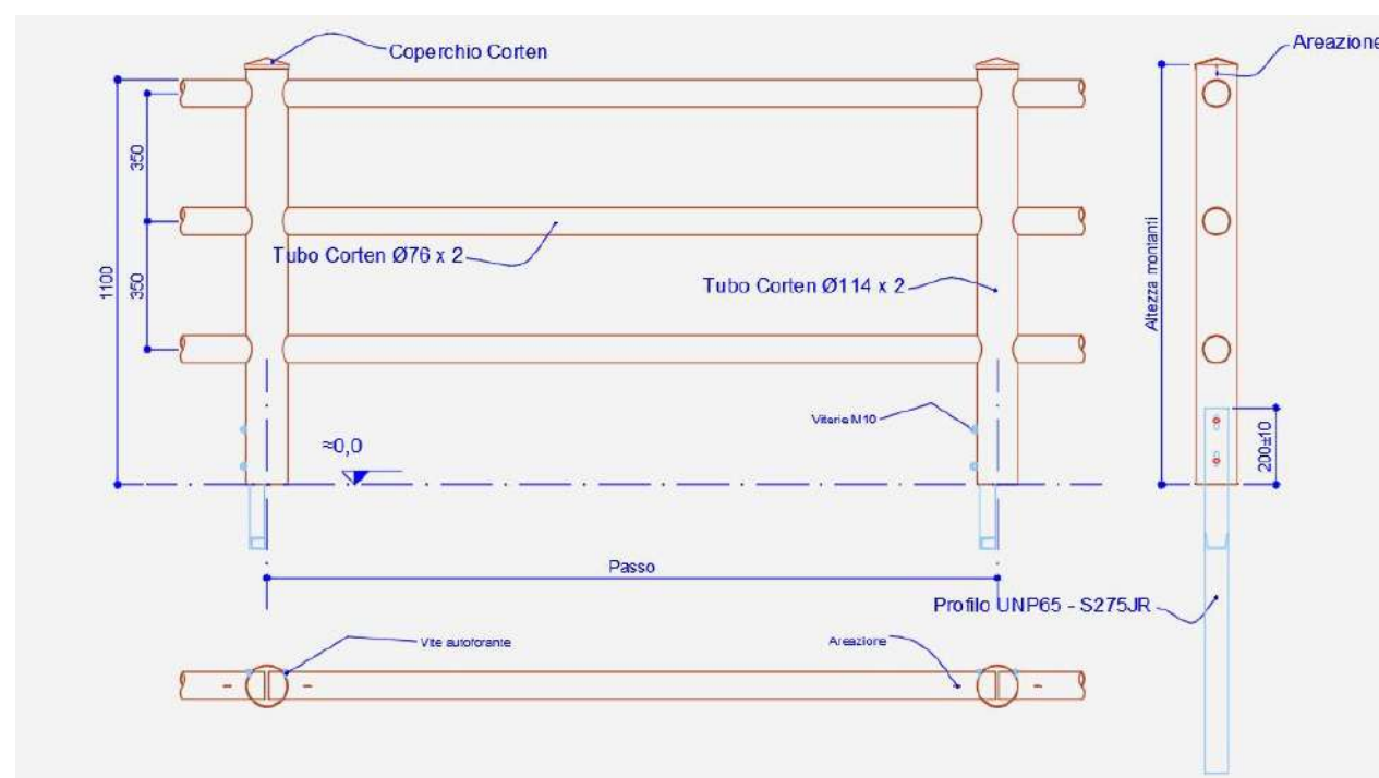
Barriera corten
