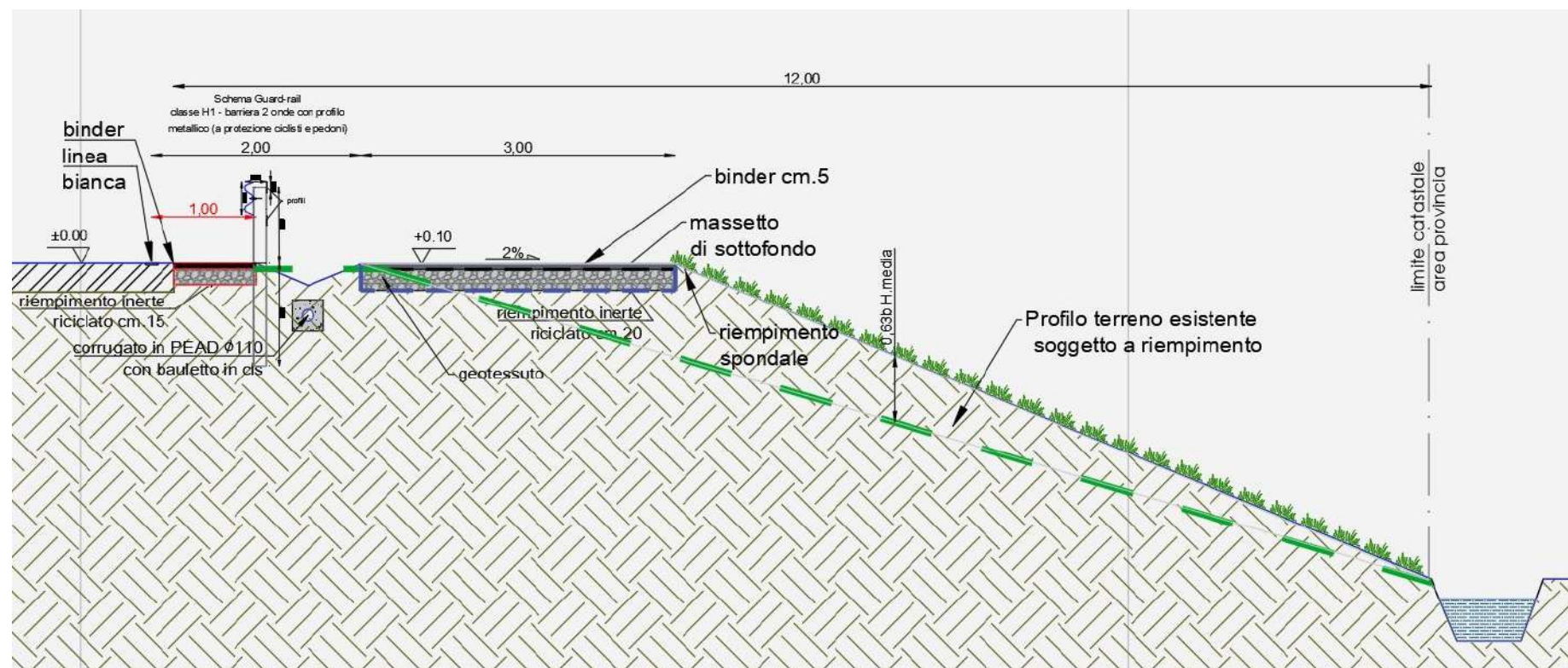
Sezione tipo percorso (tratto 3-5)
