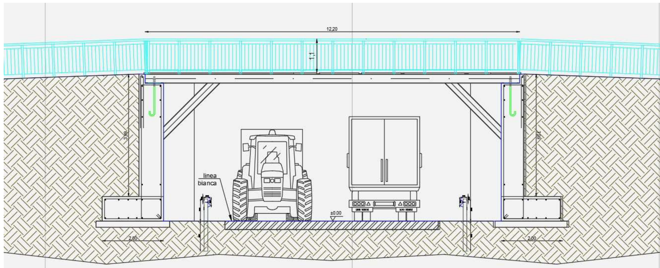
Sezione tipo percorso (tratto 4)
